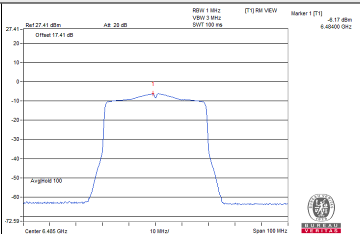
802.11ax (HE40) Beamforming / Chain 0 : CH 107
