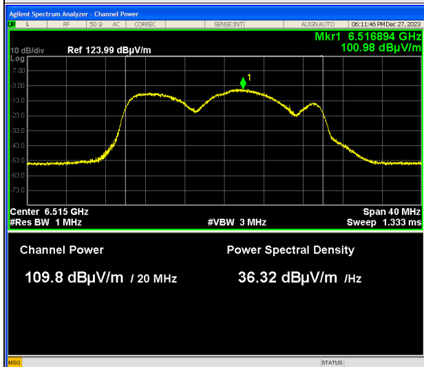
802.11ax (HE20) CDD : CH 113
