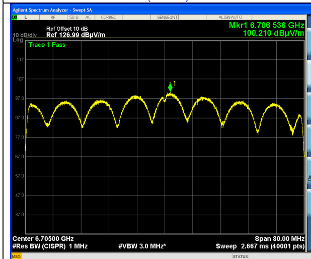
802.11ax (HE80) CDD : CH 151
