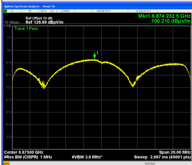
802.11ax (HE20) CDD : CH 185
