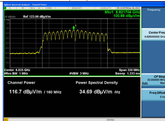
802.11ax (HE160) CDD : CH 175
