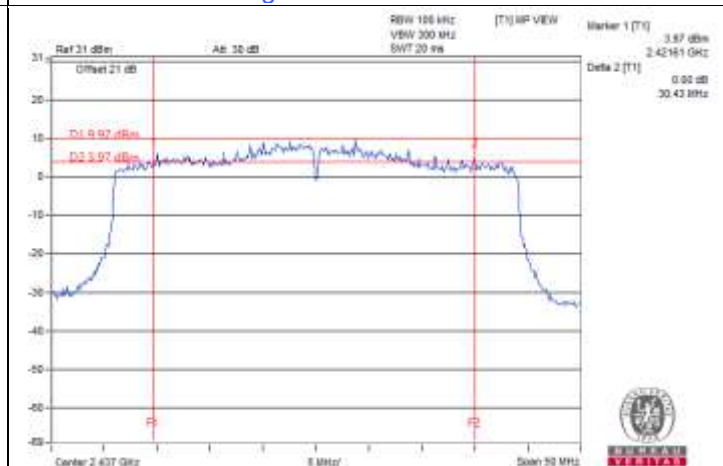
802.11ax (HE40) CDD / Chain 0 : CH 6
