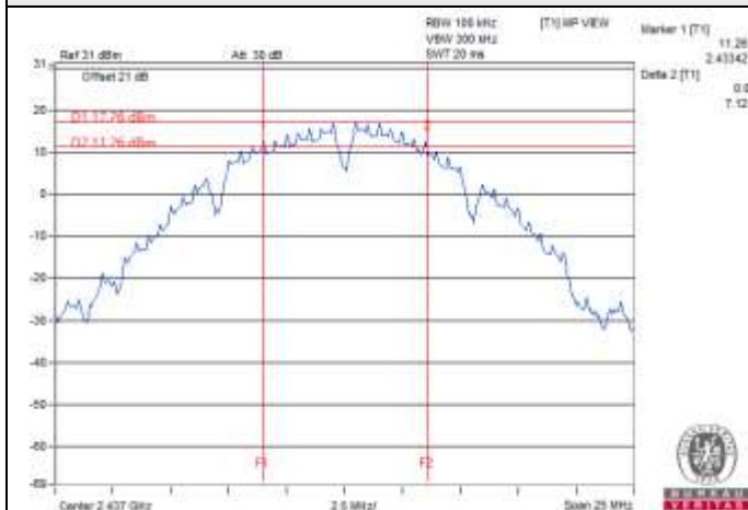
802.11b CDD / Chain 1 : CH 6
