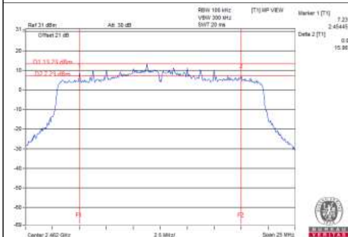
802.11ax (HE20) CDD / Chain 1 : CH 11
