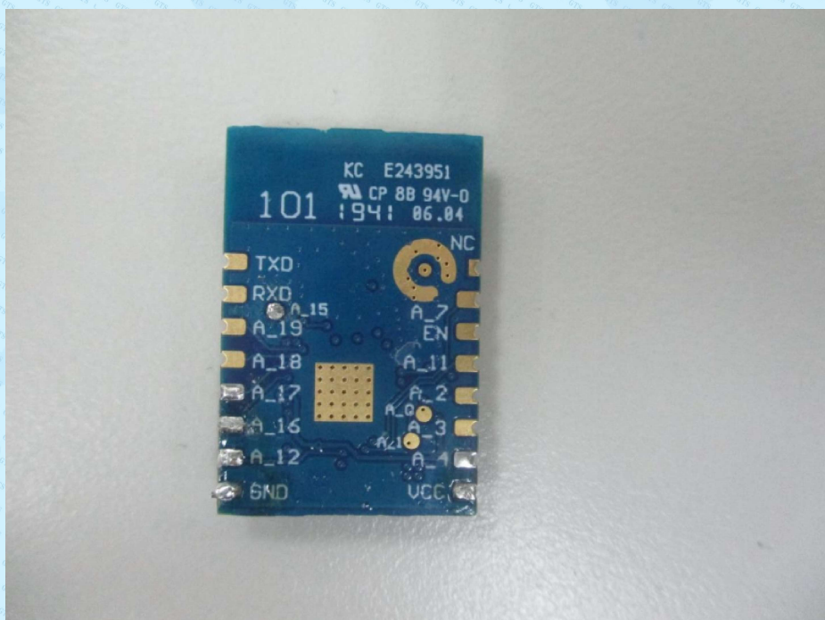
EUT Photo
