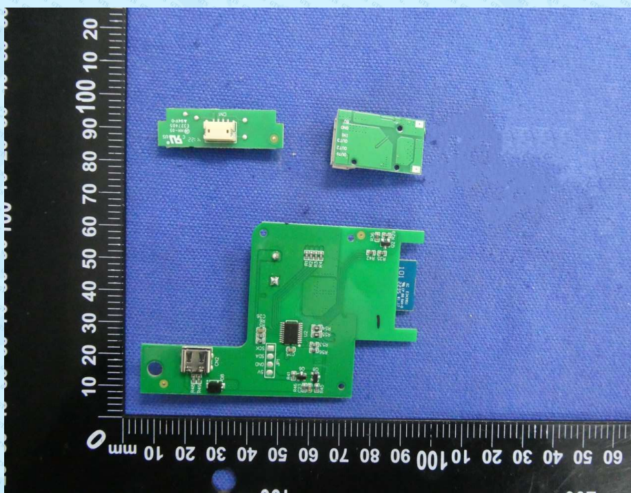
EUT Photo
