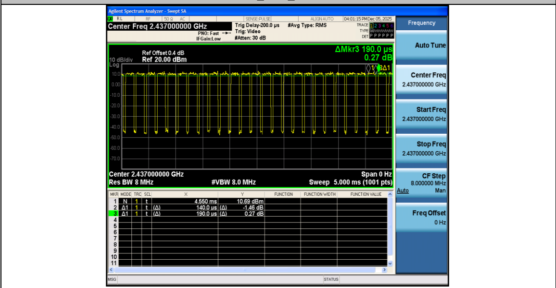
11G_Ant2_2437
