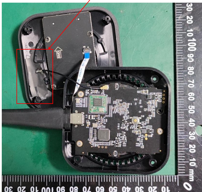
antenna
