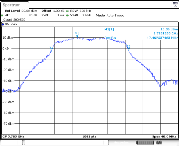
11A Ant0 5785
