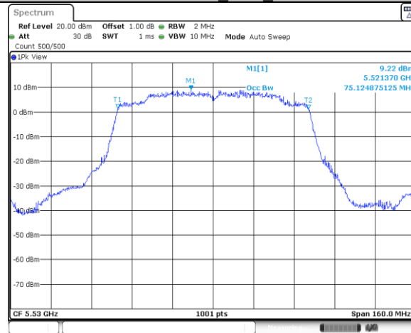
11AC80SISO Ant0 5530
