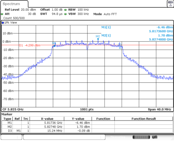
11A_Ant1_5825
