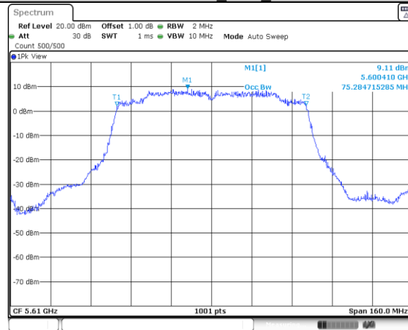
11AC80SISO Ant0 5610
