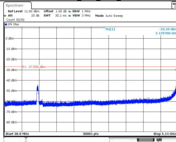
11AC80SISO Ant0 5210 30~5140
