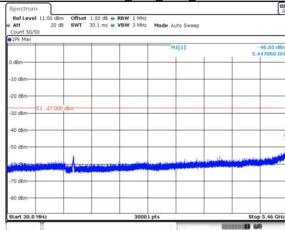
11AC40SISO Ant0 5510 30~5460
