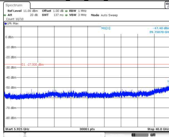
11N20SISO Ant1 5745 5925-40000
