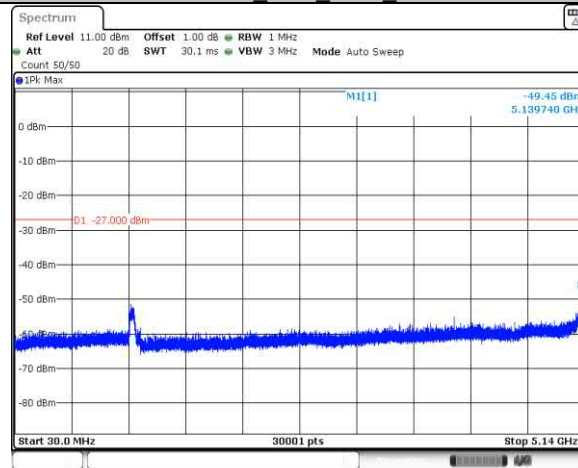
11AC80SISO Ant1 5290 30~5140
