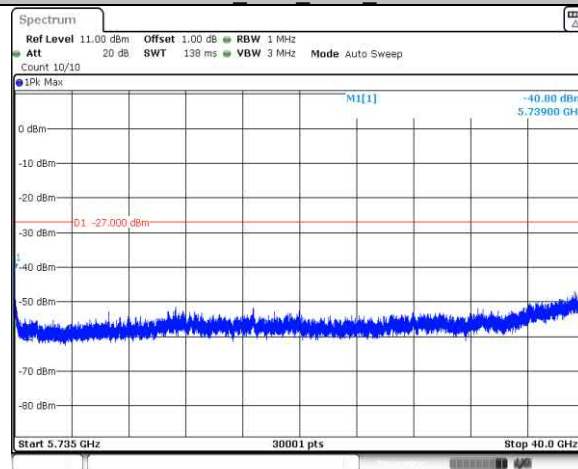
11AC20SISO Ant1 5700 5735~40000
