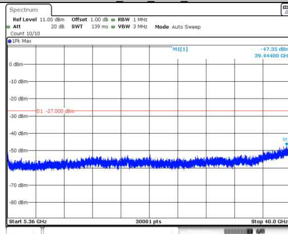
11AC80SISO Ant1 5210 5360~40000
