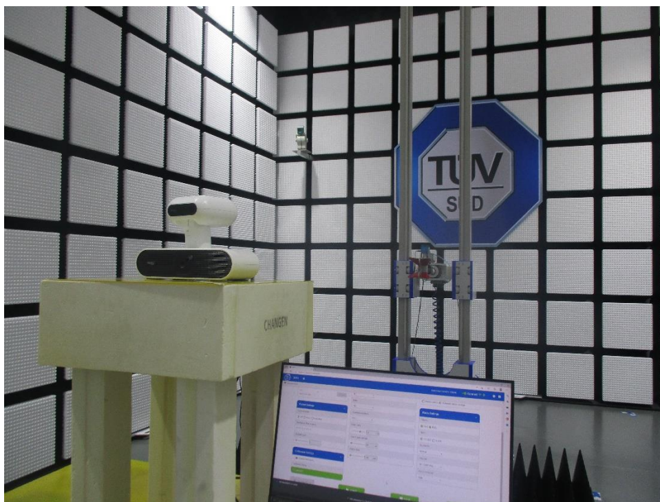
1G-18GHz RSE Setup
