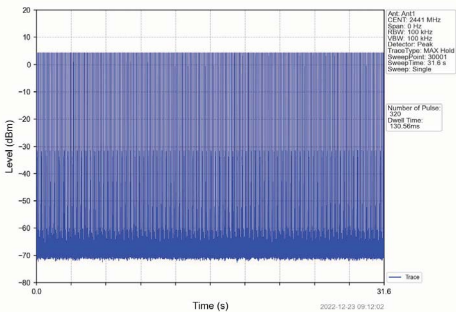
Pi/4DQPSK_2DH1_HOPP_Ant1_NTNV
