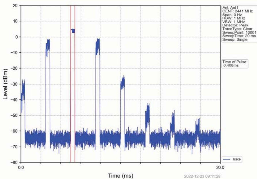
Pi/4DQPSK_2DH1_HOPP_Ant1_NTNV
