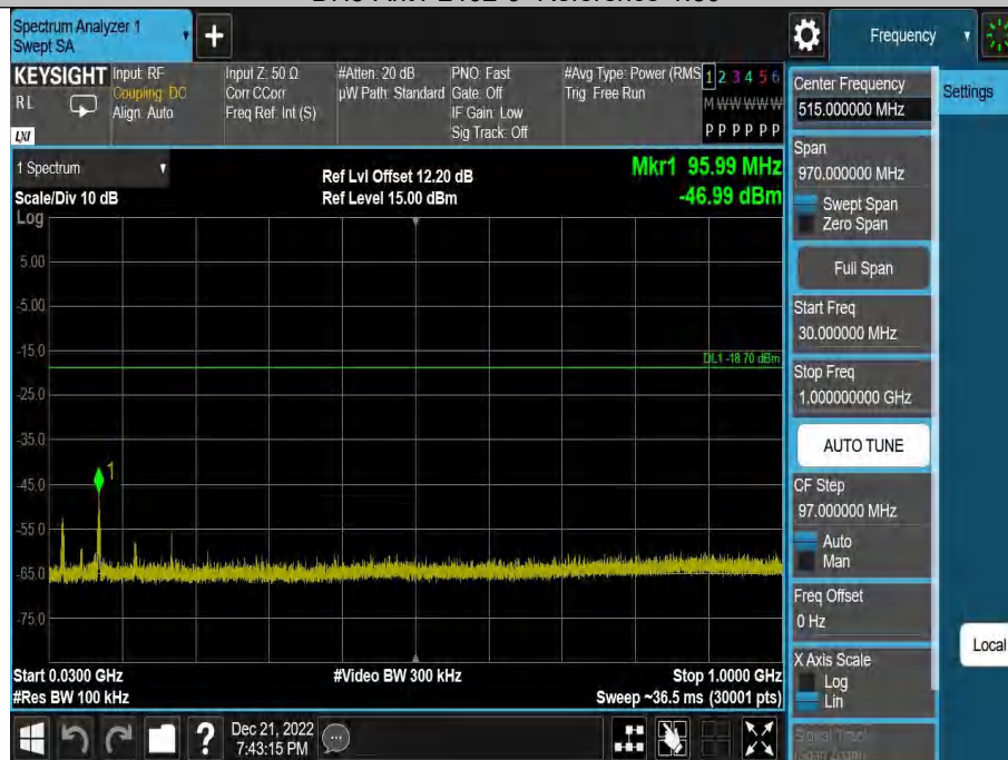
DH5-Ant1-2402-30~1000-1.30
