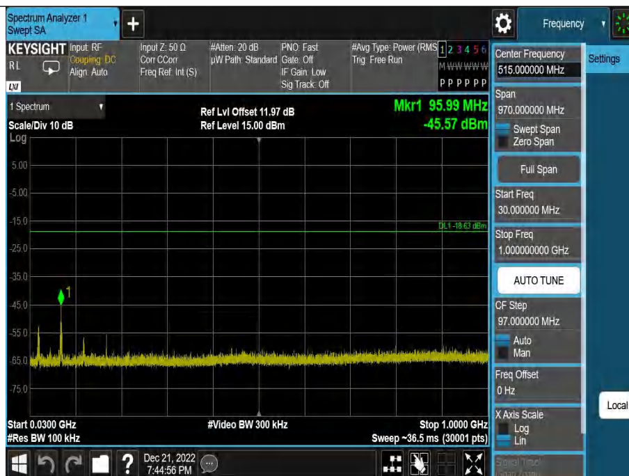
DH5-Ant1-2441-30~1000-1.37
