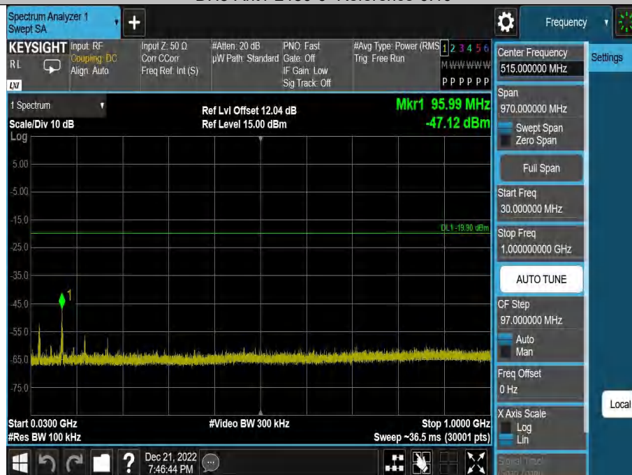
DH5-Ant1-2480-30~1000-0.10
