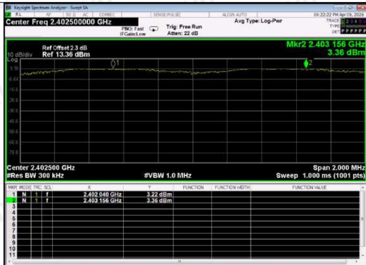
\pi/4 DQPSK
