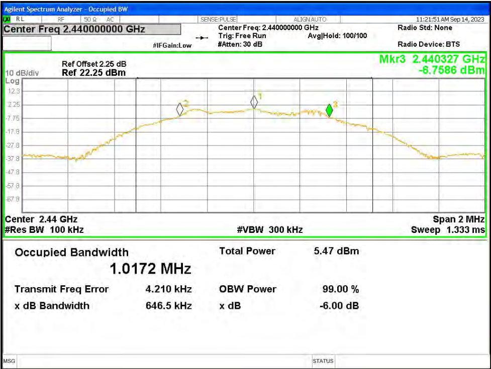
-6dB Bandwidth NVNT BLE 1M 2440MHz Ant3
