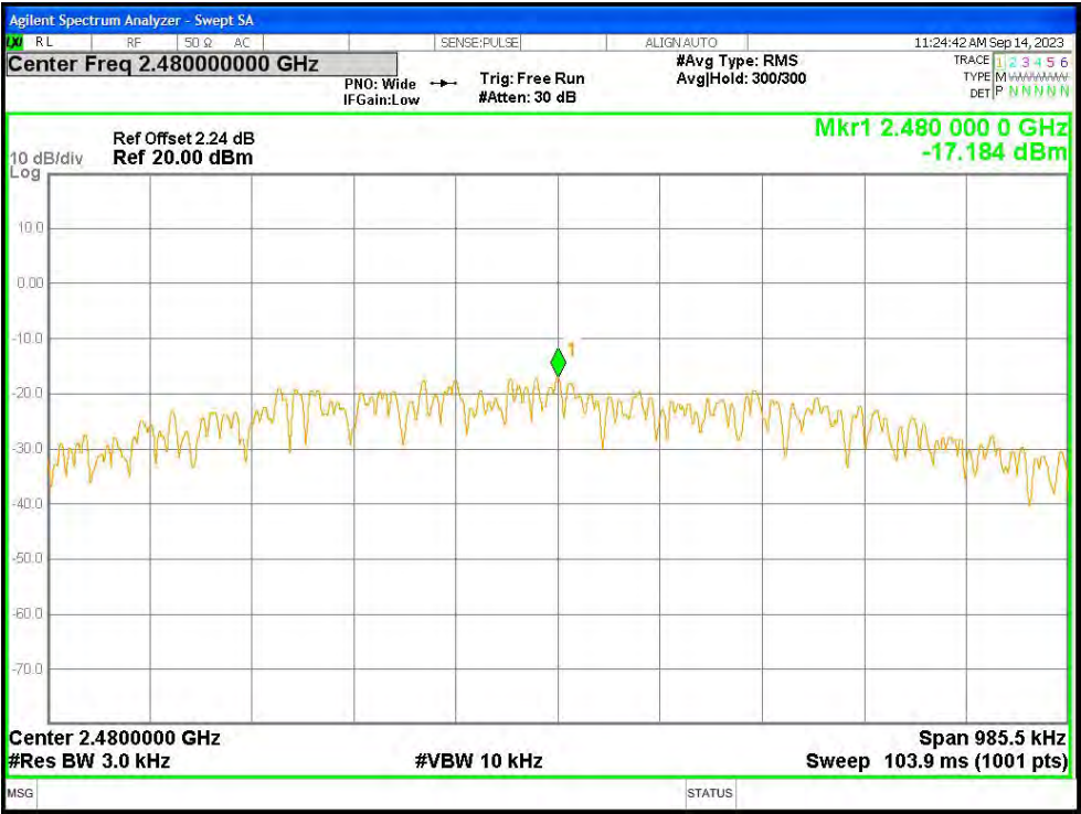
PSD NVNT BLE 1M 2480MHz Ant3
