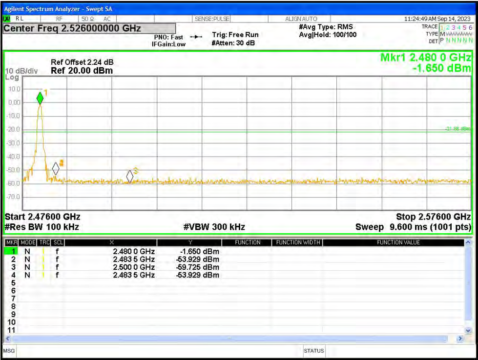
Band Edge NVNT BLE 1M 2480MHz Ant3 Emission
