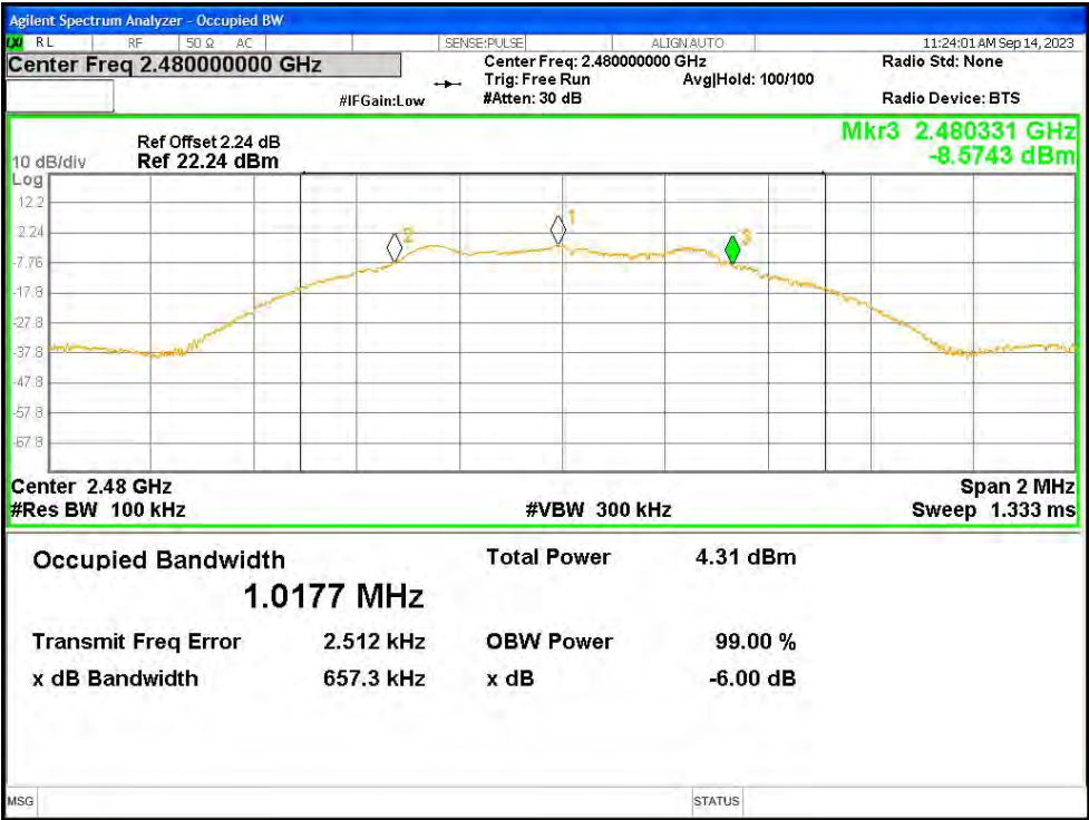
-6dB Bandwidth NVNT BLE 1M 2480MHz Ant3
