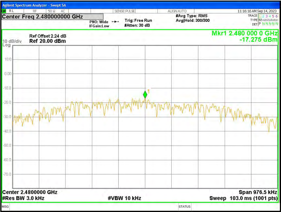
PSD NVNT BLE 1M 2480MHz Ant2
