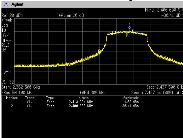
802.11n Ch 1 Band edge
