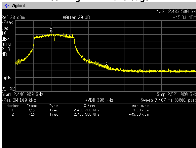
802.11g Ch 11 Band edge
