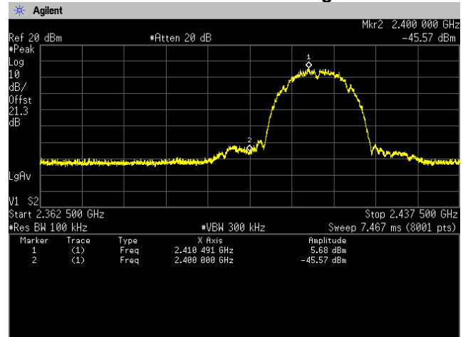
802.11b Ch 1 Band edge
