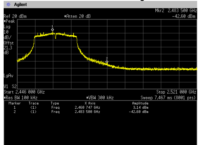
802.11n Ch 11 Band edge
