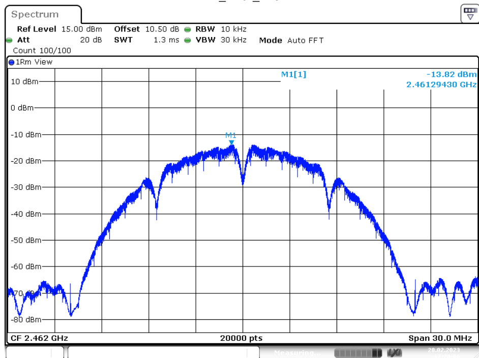
11B_Ant1_2462
