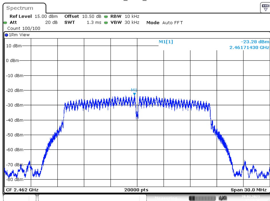
11G_Ant1_2462
