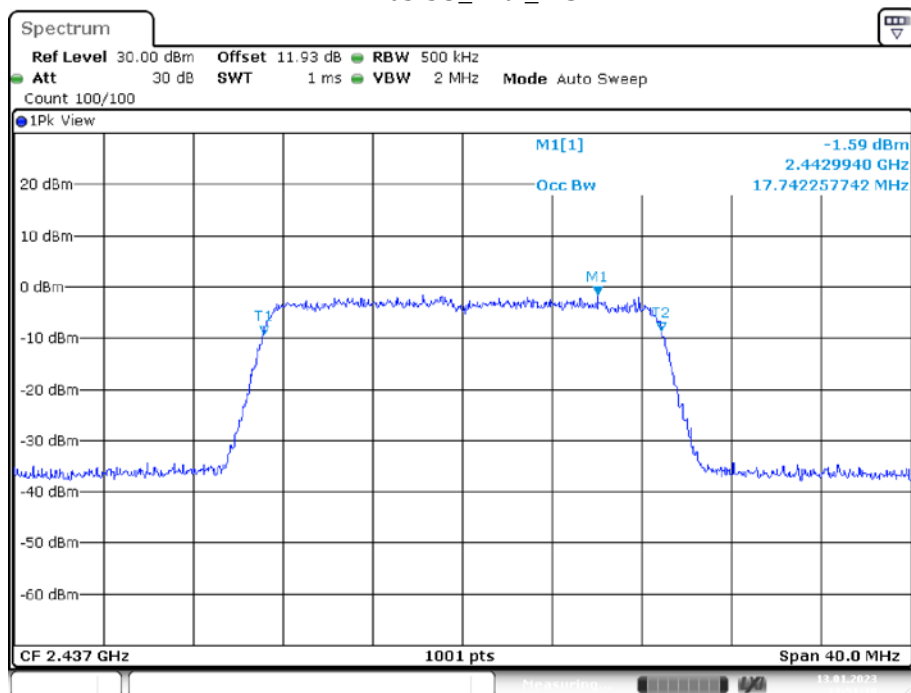
11N20SISO_Ant1_2437
