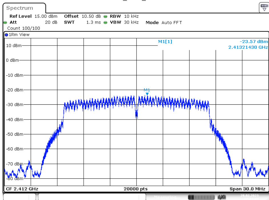
11G_Ant1_2412
