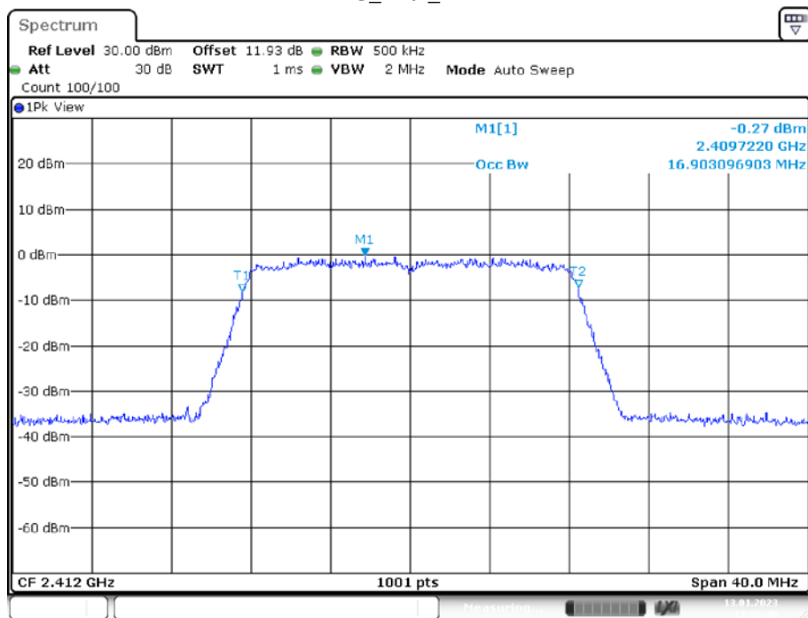
11G_Ant1_2412
