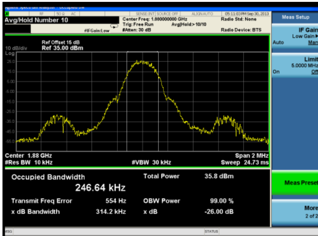
(Plot K: GSM 1900MHz Channel = 661)
