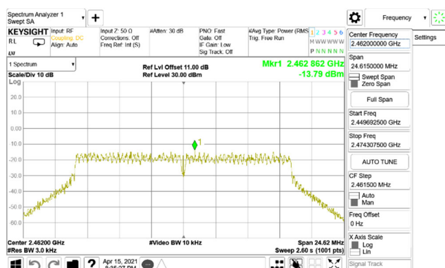
802.11g_20MHz_Chain0_2462MHz
