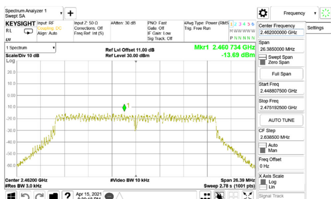
802.11n_20MHz_Chain0_2462MHz
