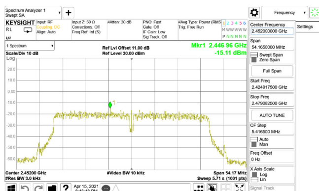
802.11n_40MHz_Chain0_2452MHz
