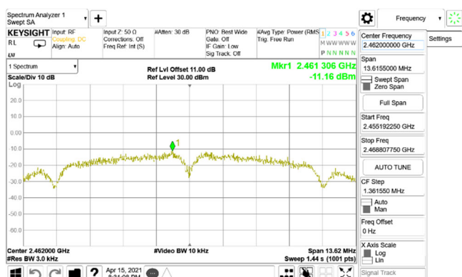
802.11b_20MHz_Chain0_2462MHz
