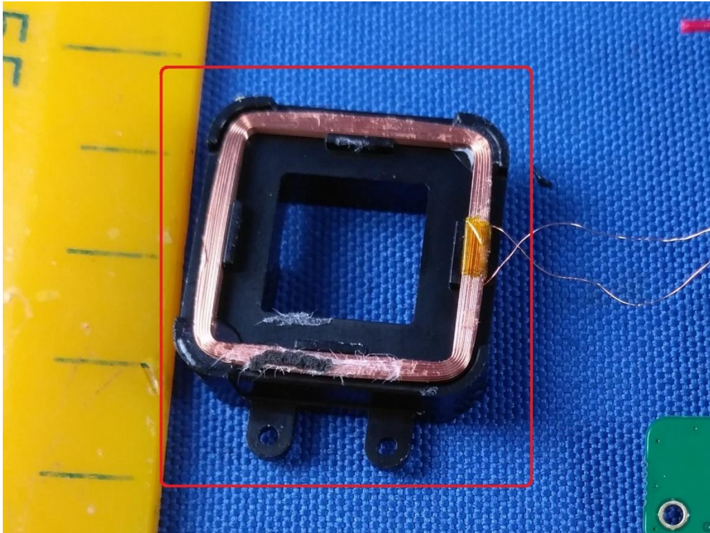
RFID Antenna
