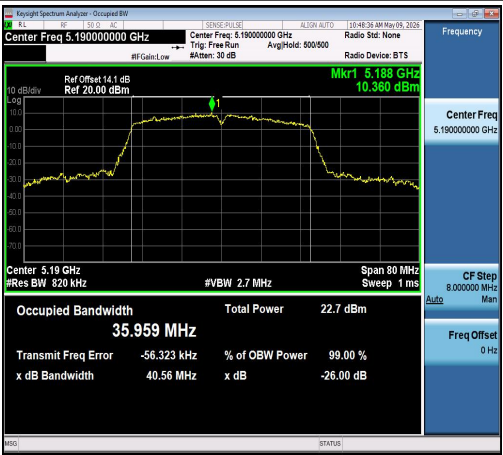
11N40MIMO-Ant0-5190
