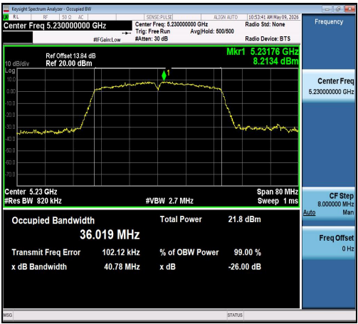
11N40MIMO-Ant1-5230
