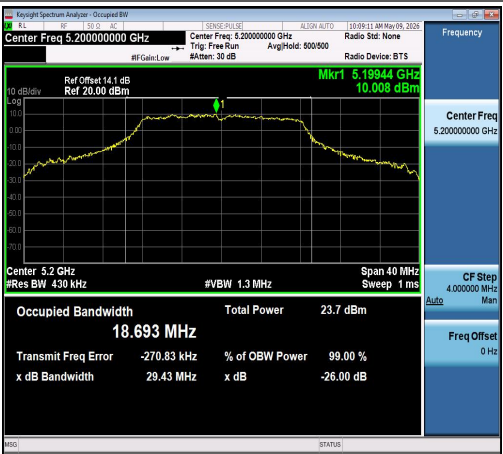
11A-Ant0-5200
