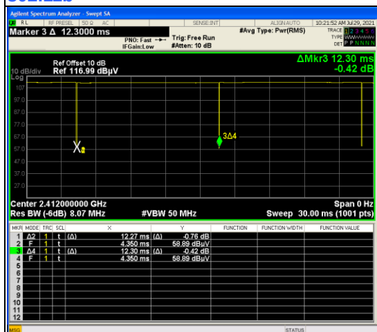
802.11n (HT20)
