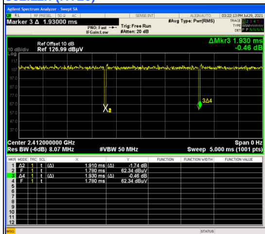
802.11n (HT20)
