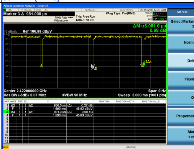
802.11n (HT40)
