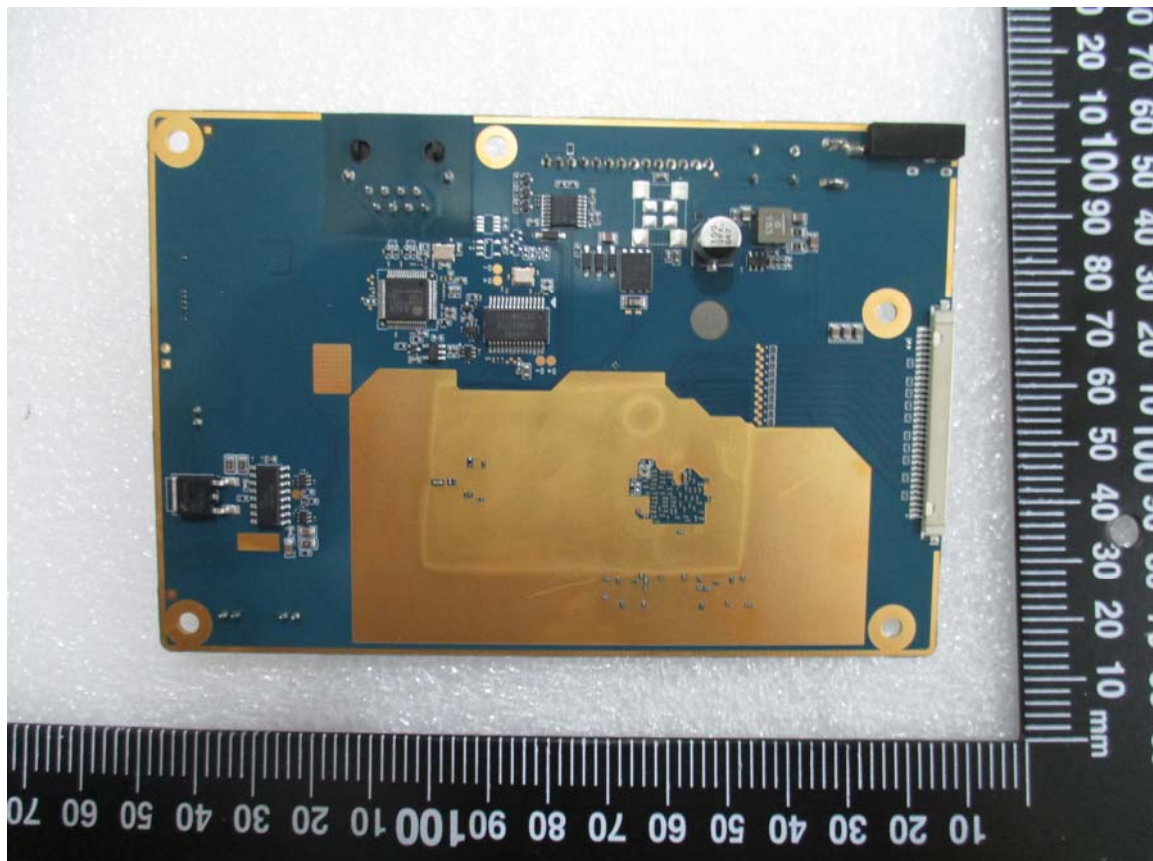
WiFi+BT+ANT+ module
