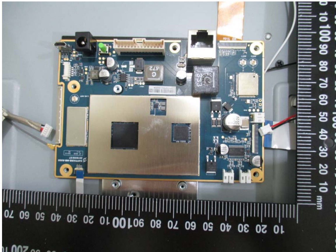
WiFi+BT+ANT+ module
