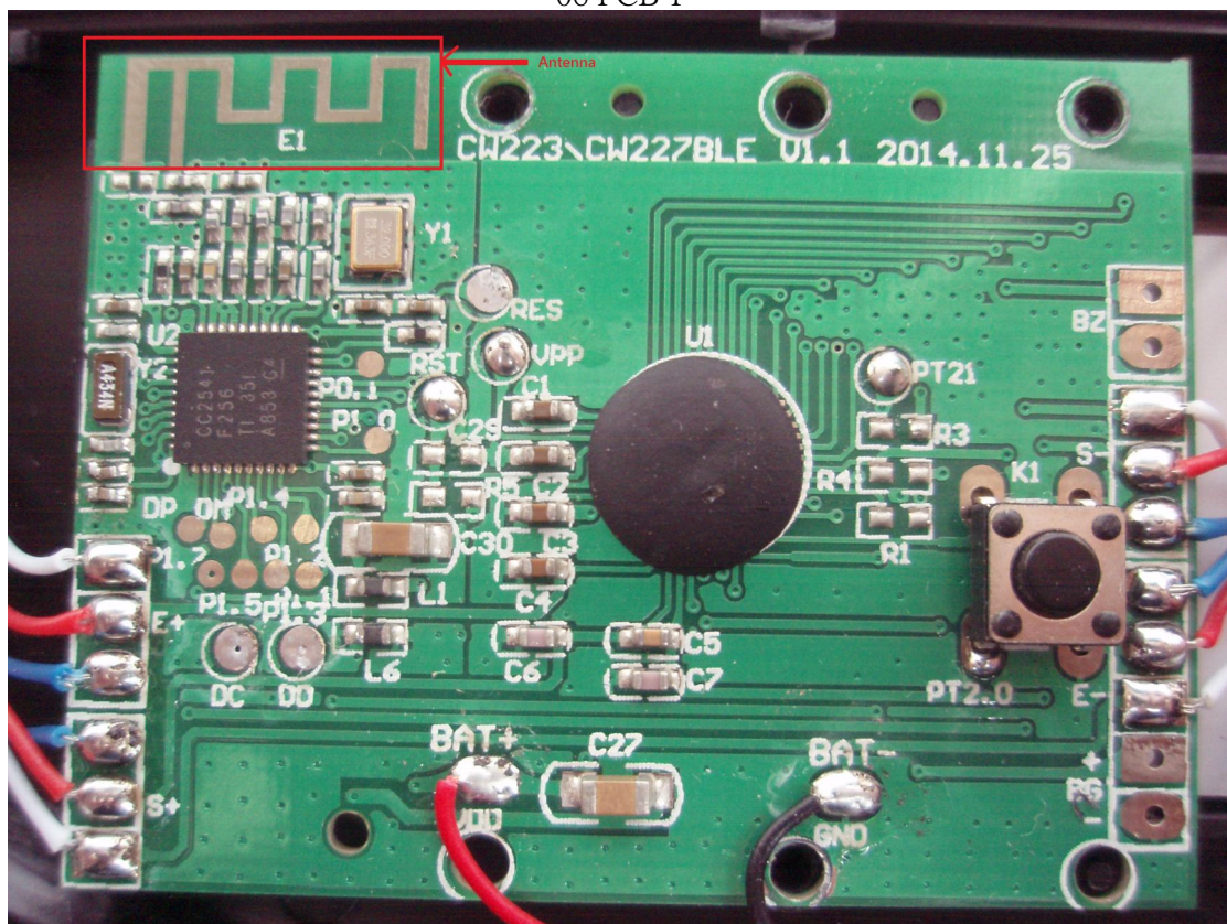
06 PCB-F
