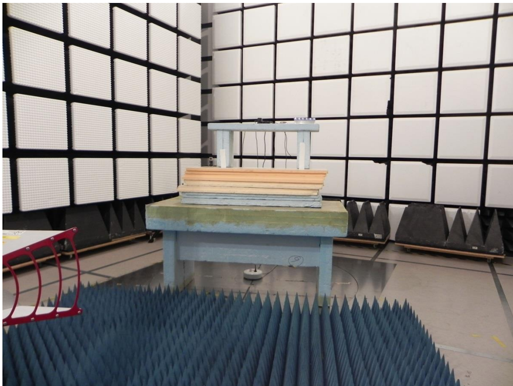
EUT 1: 1-8.2 GHz:
