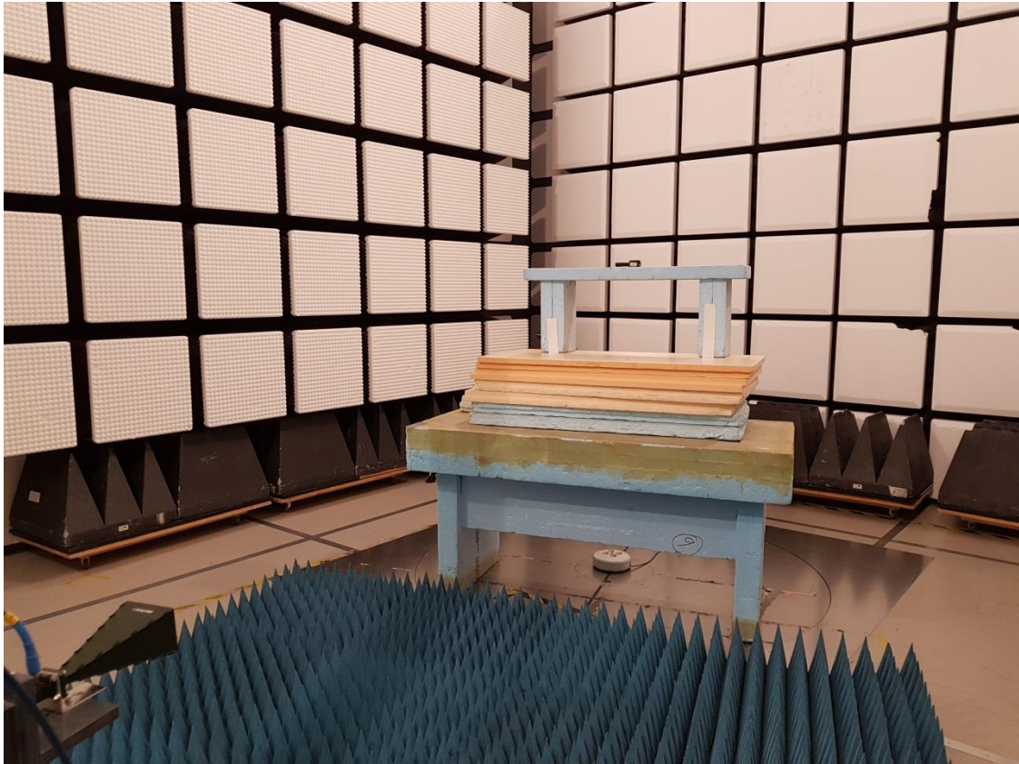
EUT 2, Y-axis: 8.2-18 GHz:
