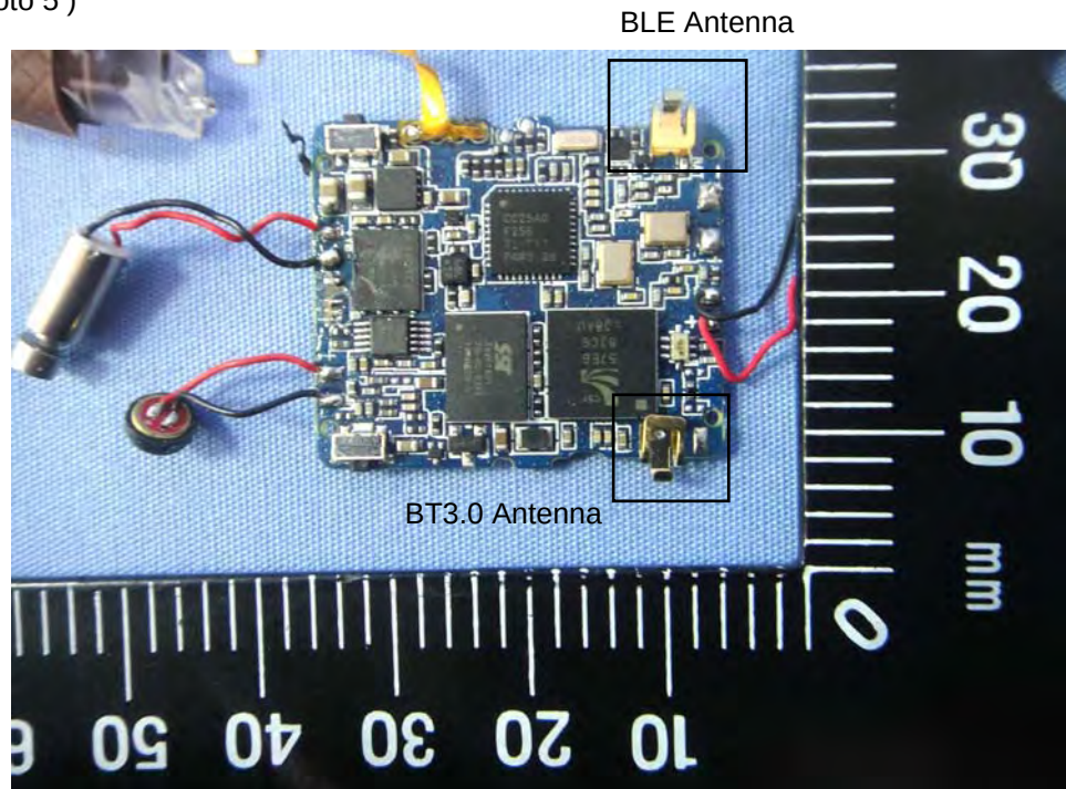
EUT Photo 6 )
