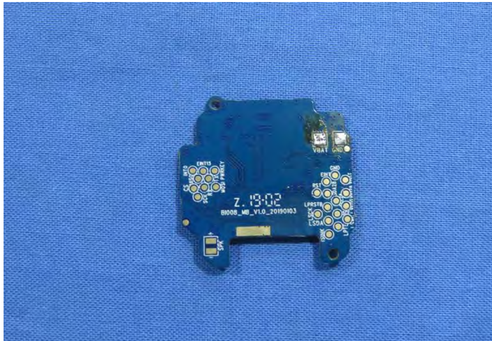
EUT Photo (12)
