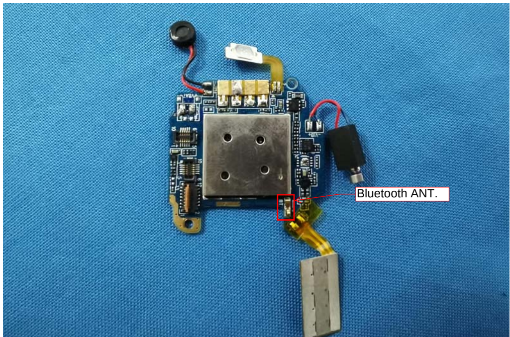
EUT Photo (10)
