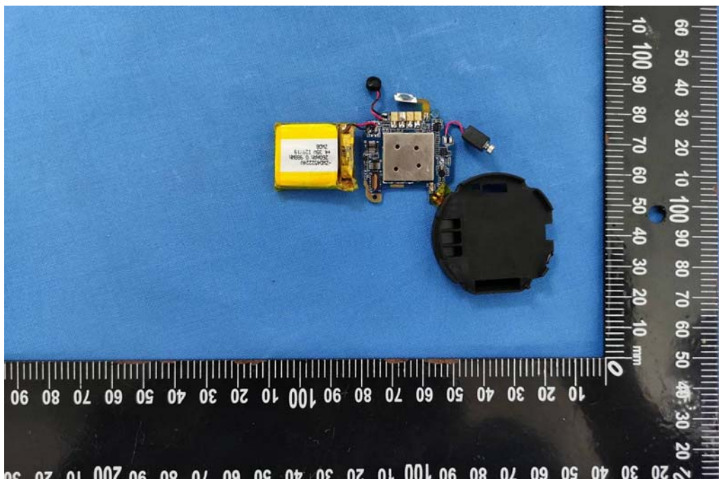
EUT Photo (6)
