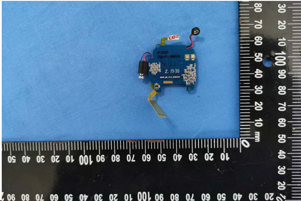
EUT Photo (8)
