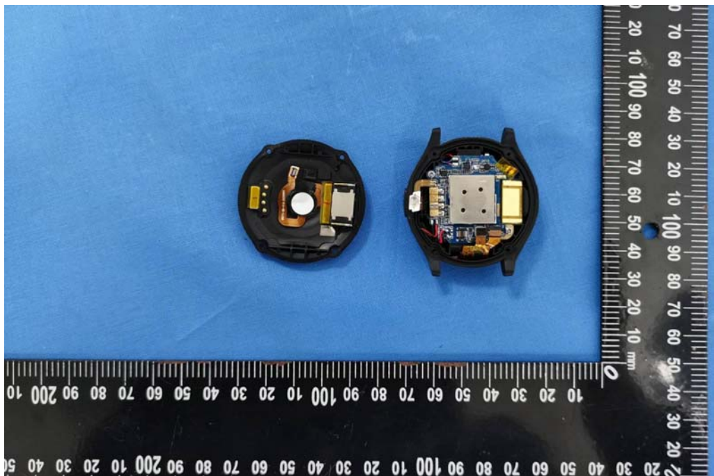
EUT Photo (2)
