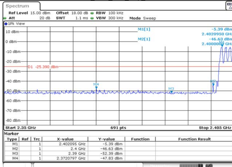
DH5_Ant1_Low_Hop_2402
