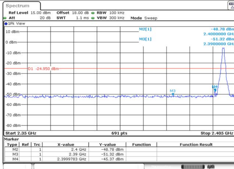
DH5_Ant1_Low_2402
