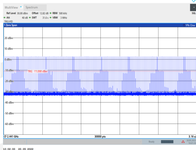
2DH5_Ant1_Hop
