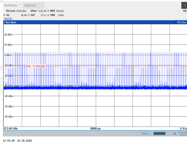
3DH1_Ant1_Hop
