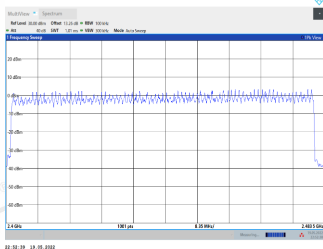
3DH5_Ant1_Hop
