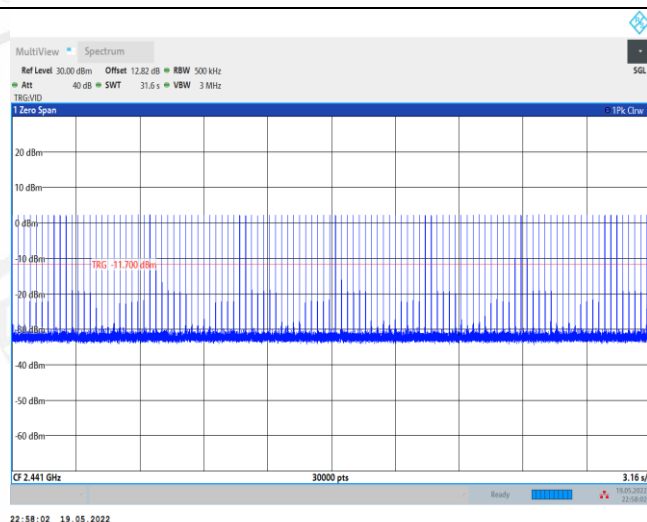
2DH1_Ant1_Hop
