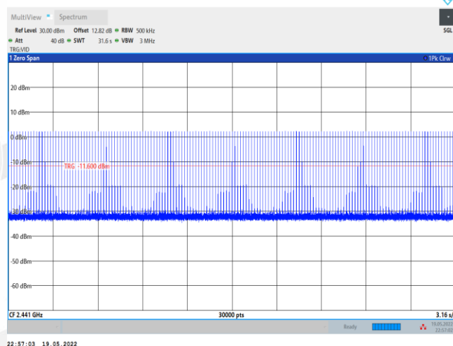
DH5_Ant1_Hop
