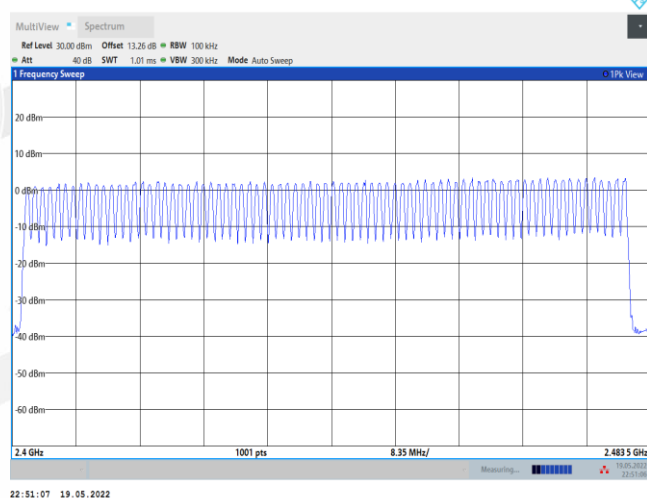
2DH5_Ant1_Hop
