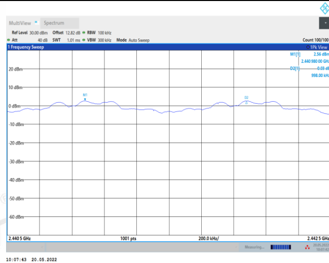
3DH5_Ant1_Hop
