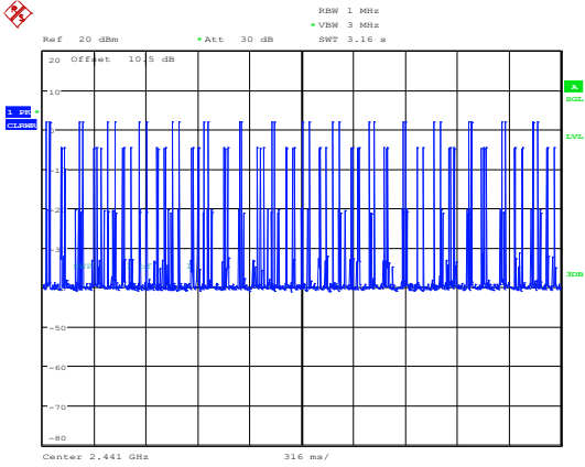
DH1_Hopping
