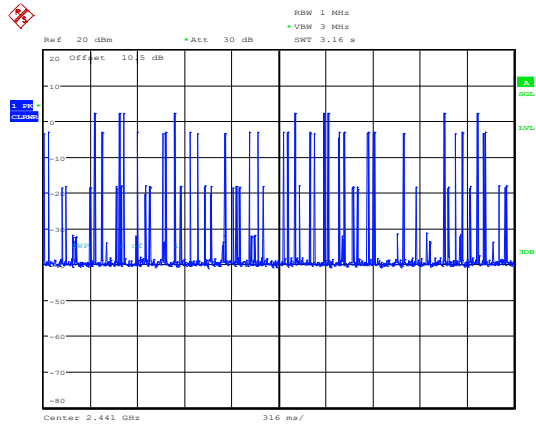
2DH5_Hopping
