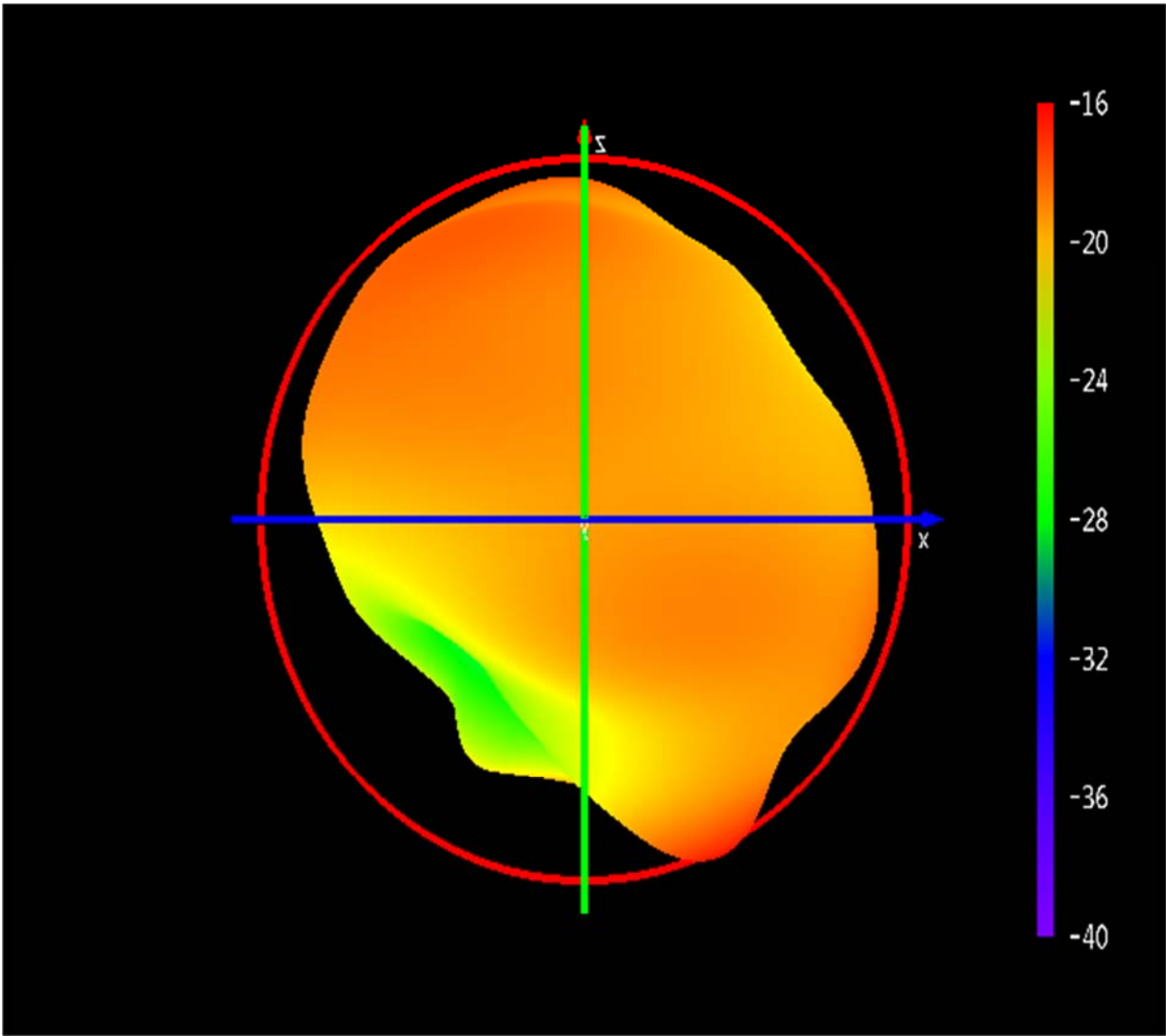
2402MHZ
