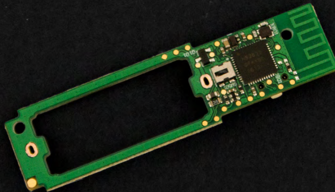
FGBHDW-002 PCB View „A”
