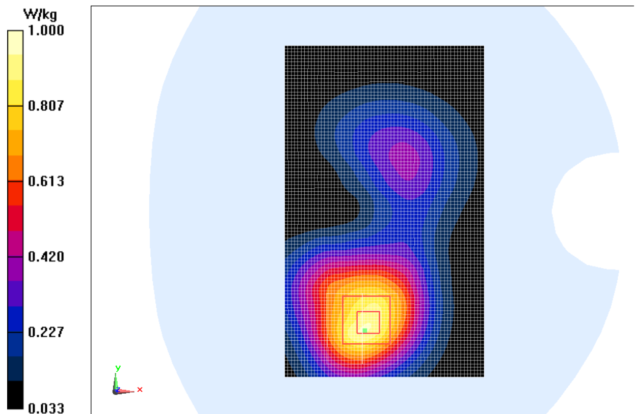
Fig.8 WCDMA1900 CH9538
