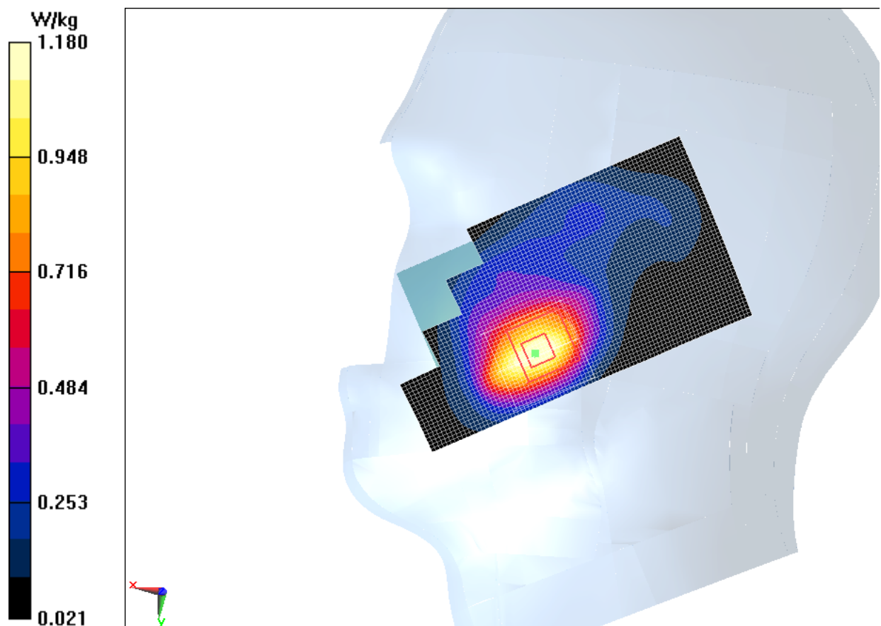
Fig.7 WCDMA1900 CH9538
