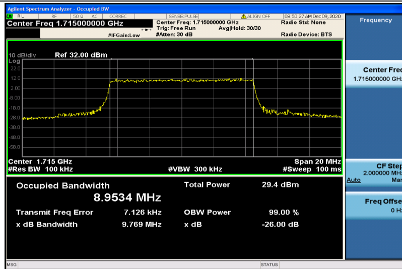
Band66-10MHz-QPSK-132022-50RB#0-8.9534
