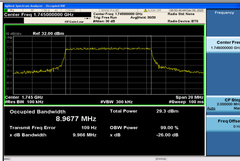
Band66-10MHz-QPSK-132322-50RB#0-8.9677
