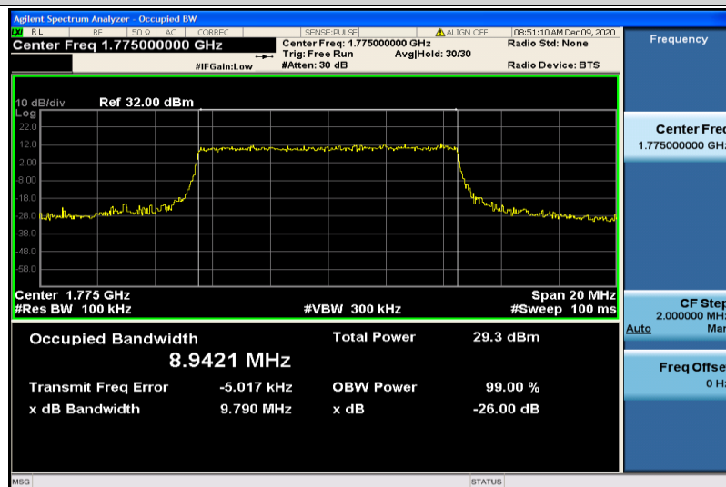
Band66-10MHz-QPSK-132622-50RB#0-8.9421
