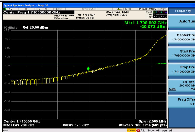
Band66-20MHz-QPSK-132072-1RB#0
