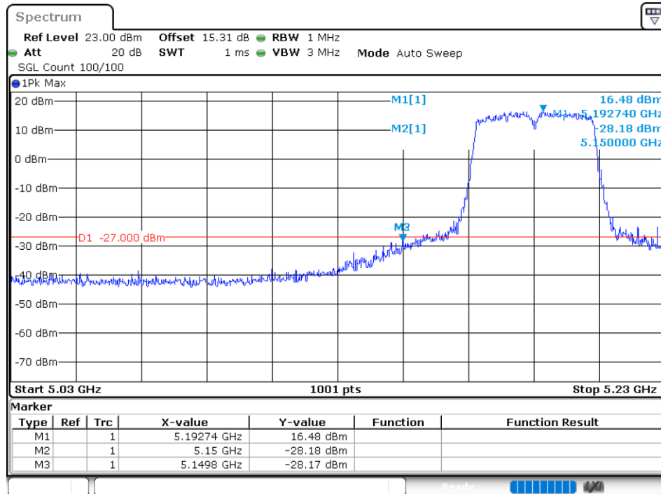
Band Edge NVNT n40 5230MHz High Ant 4
