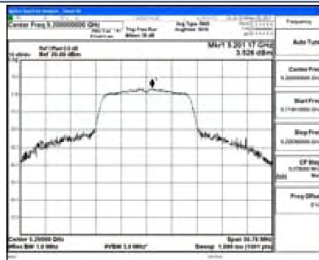
802.11n(HT20)-5200MHz
