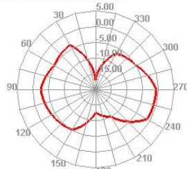
2440.000MHz E2
