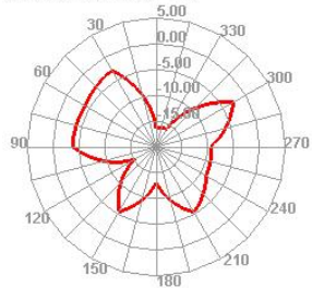
2480.000MHz E1
