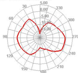
2440.000MHz E2
