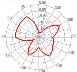
2440.000MHz E1
