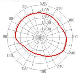
2440.000MHz H
