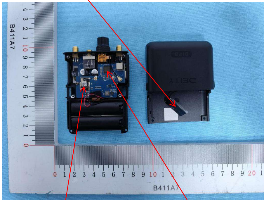
BLE RF IC 2: TSLR8258F512ET32
