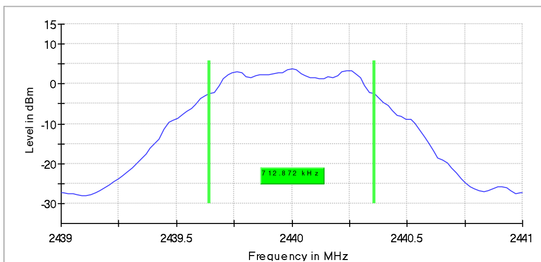
BLE 1M Ant1 2440
