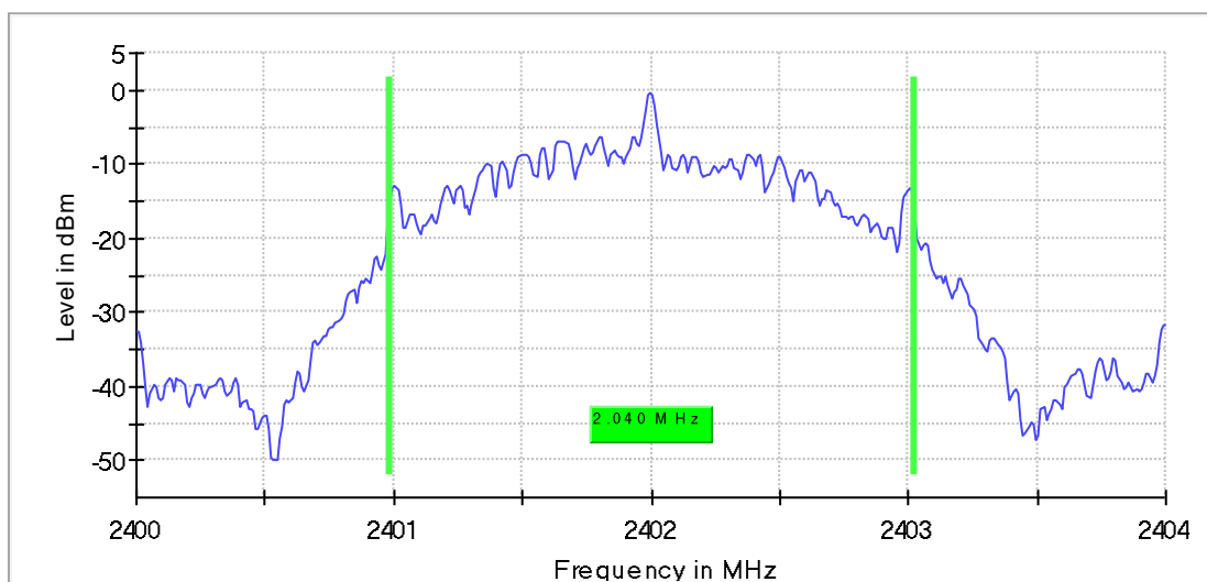
BLE 2M Ant1 2402
