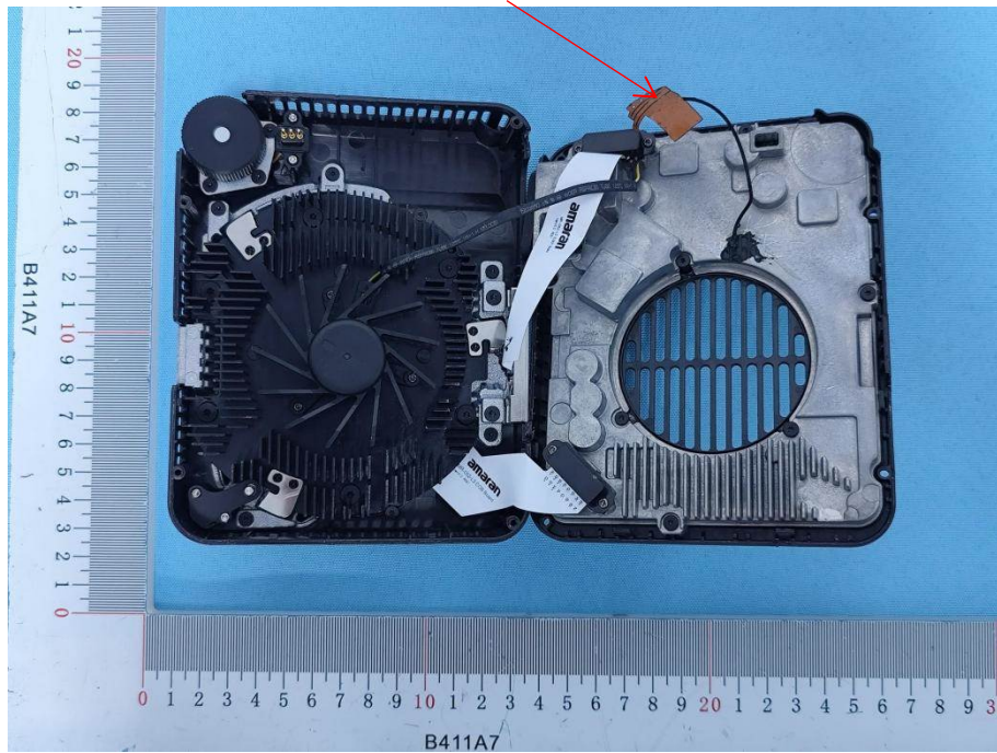
NFC RX ANT
