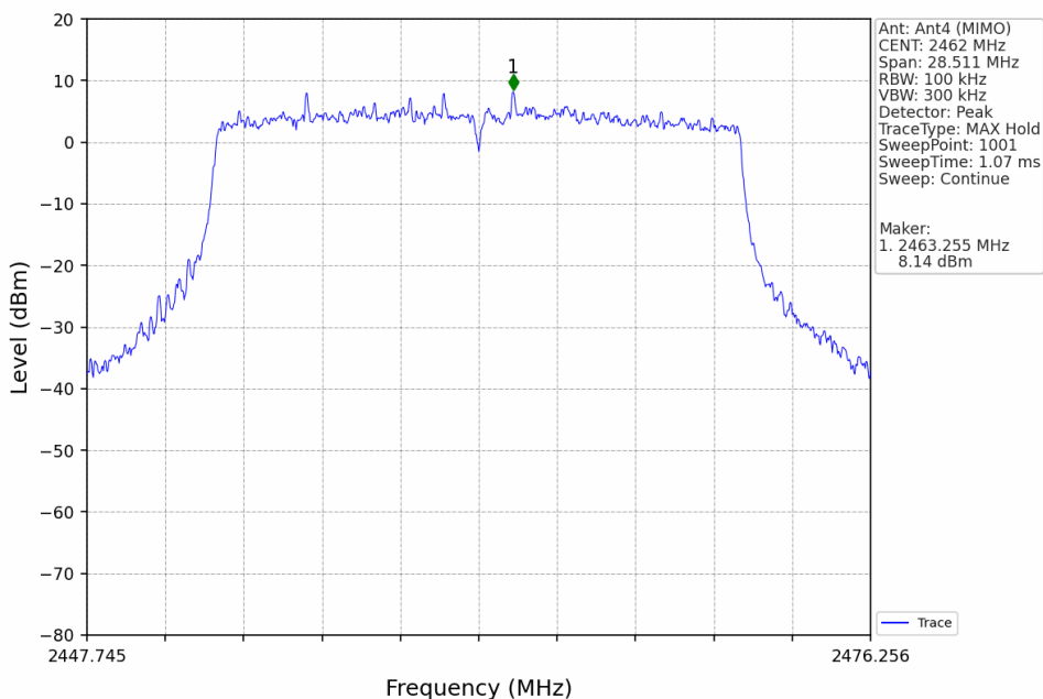
802.11ax(HEW20)_HCH_2462MHz_RU242_Left_Ant4 (MIMO)_NTNV
