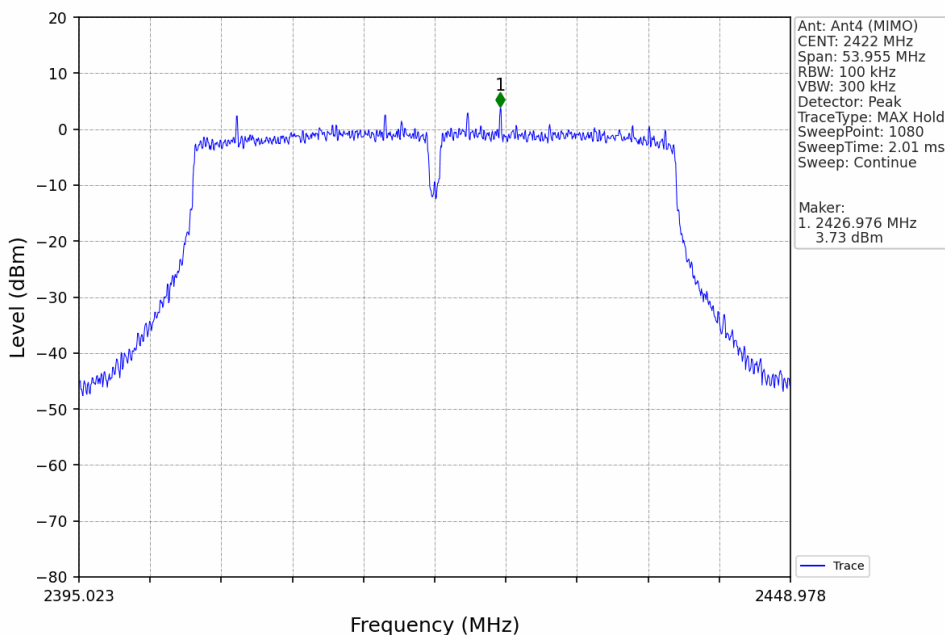
802.11n(HT40)_LCH_2422MHz_Ant4 (MIMO)_NTNV
