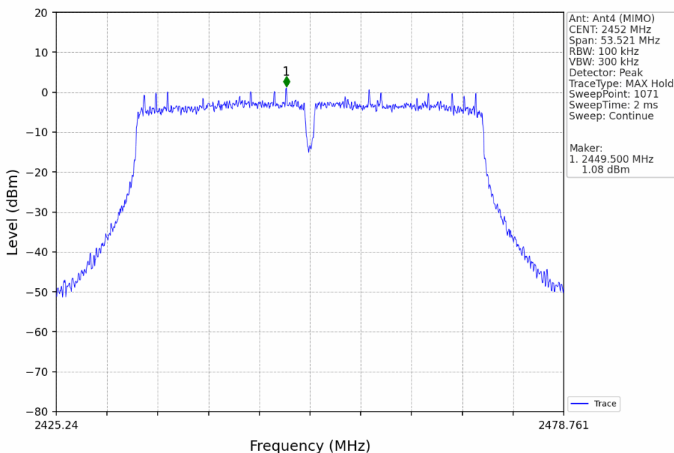
802.11n(HT40)_HCH_2452MHz_Ant4 (MIMO)_NTNV
