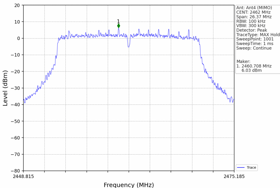
802.11n(HT20)_HCH_2462MHz_Ant4 (MIMO)_NTNV
