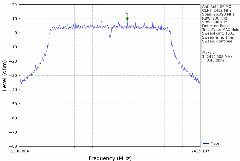
802.11n(HT20)_LCH_2412MHz_Ant4 (MIMO)_NTNV
