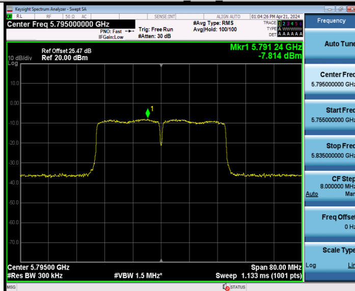
11AC80MIMO_Ant8_5210
