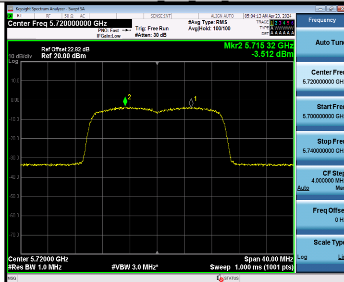
11AX20MIMO_Ant8_5720_UNII-3
