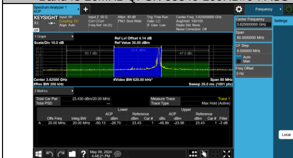
Band48-20MHz-QPSK-55990-1RB#99-PASS
