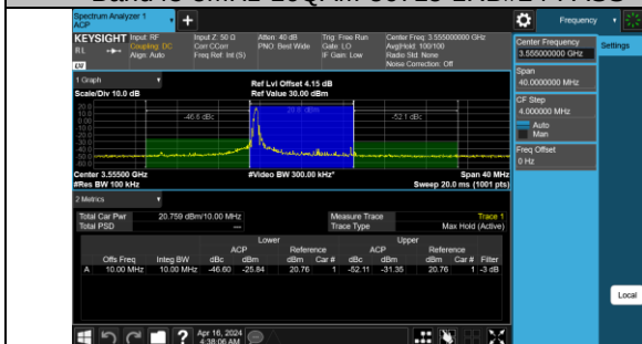
Band48-10MHz-QPSK-55290-1RB#0-PASS
