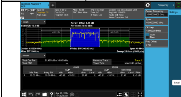
Band48-10MHz-QPSK-55290-50RB#0-PASS
