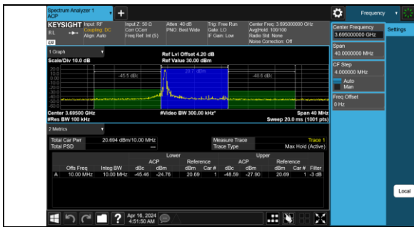
Band48-10MHz-QPSK-56690-1RB#0-PASS
