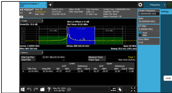
Band48-20MHz-QPSK-55340-1RB#0-PASS
