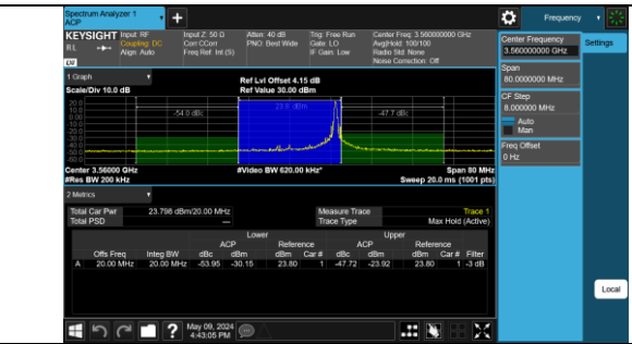
Band48-20MHz-QPSK-55340-1RB#99-PASS
