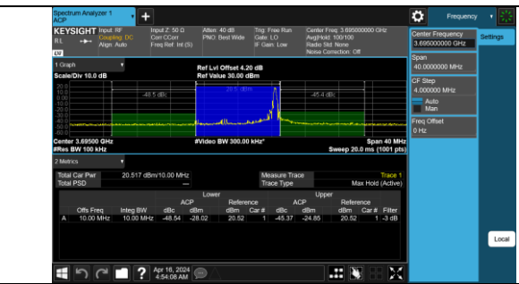
Band48-10MHz-QPSK-56690-1RB#49-PASS
