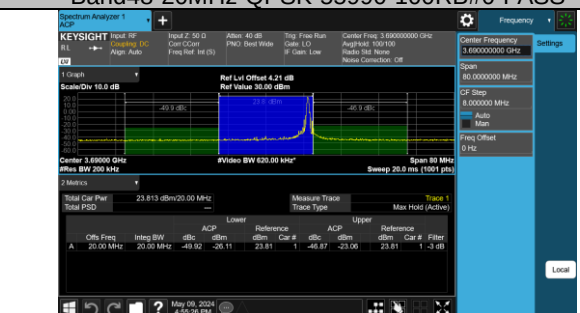
Band48-20MHz-QPSK-56640-1RB#99-PASS
