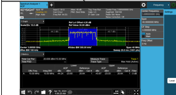
Band48-10MHz-QPSK-56690-50RB#0-PASS
