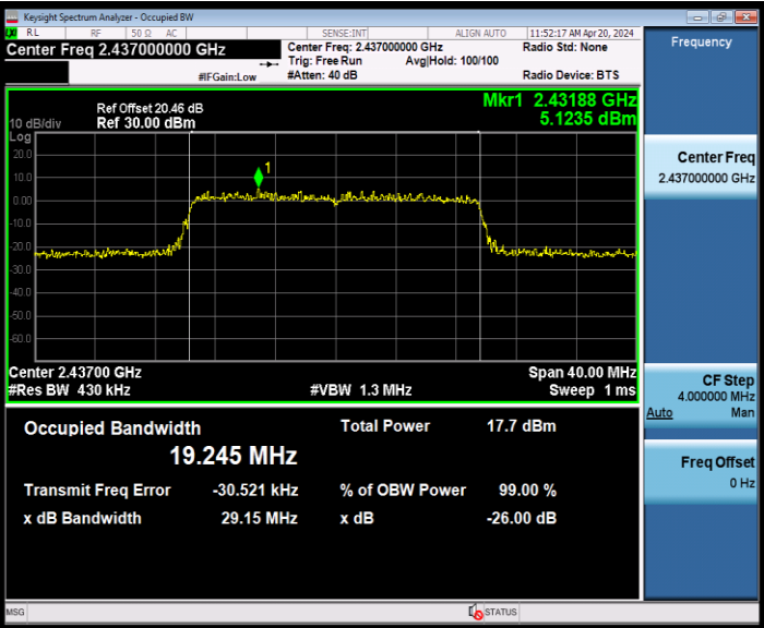
11AX20MIMO_Ant9_2437
