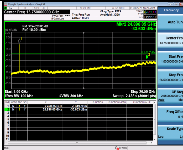
11AX40MIMO_Ant8 2437 0~Reference
