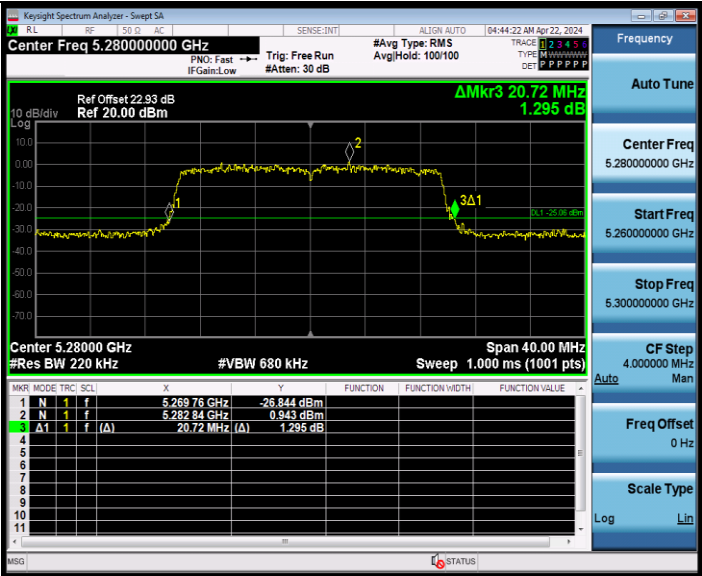
11AX20MIMO_Ant9_5280
