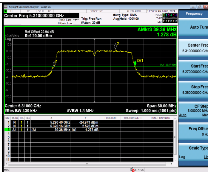
11N40MIMO Ant9 5310
