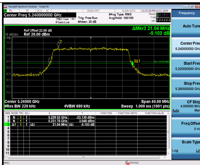
11AX20MIMO_Ant9_5240
