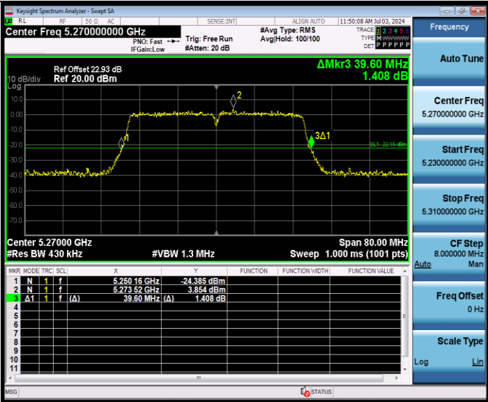
11N40MIMO Ant9 5270
