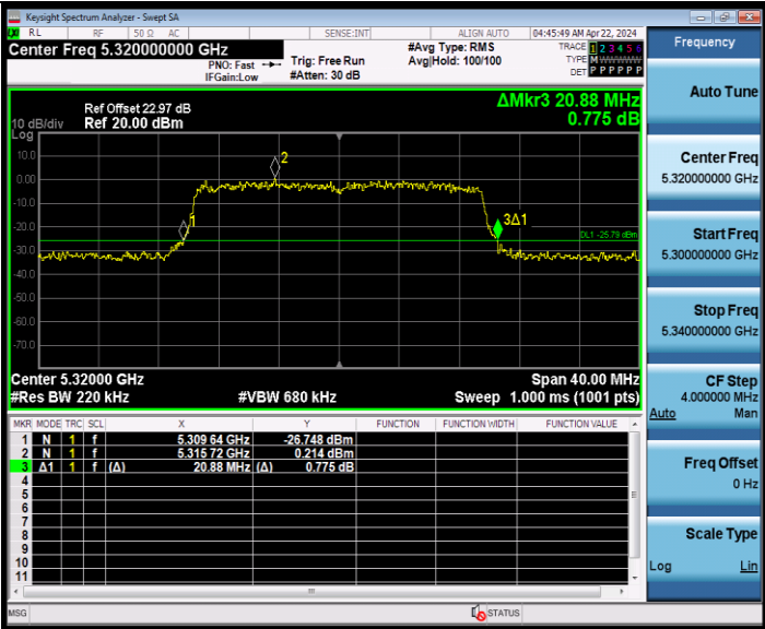
11AX20MIMO_Ant9_5320
