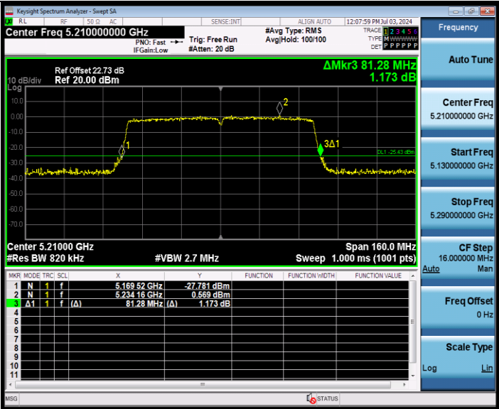
11AC80MIMO_Ant9_5210
