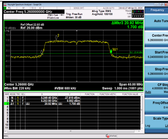
11AX20MIMO_Ant9_5260
