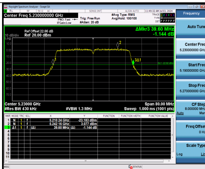
11N40MIMO Ant9 5230
