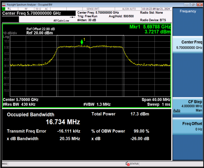
11A-CDD Ant9 5700
