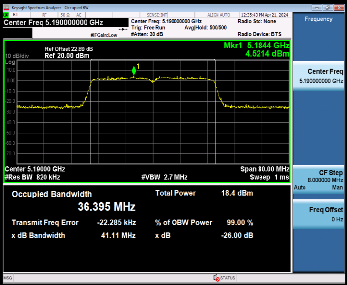
11N40MIMO_Ant9_5190
