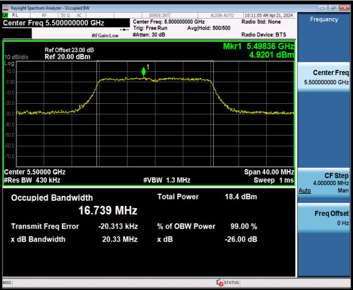
11A-CDD Ant9 5500
