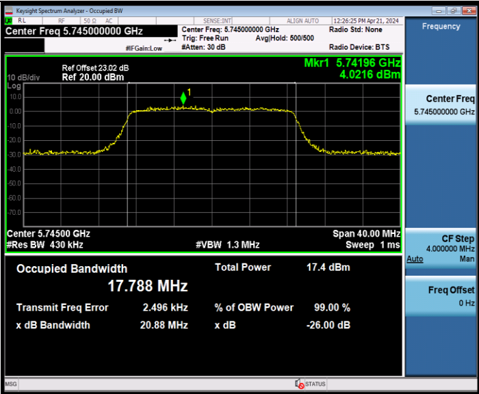
11N20MIMO_Ant9_5745
