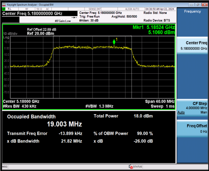
11AX20MIMO_Ant9_5180
