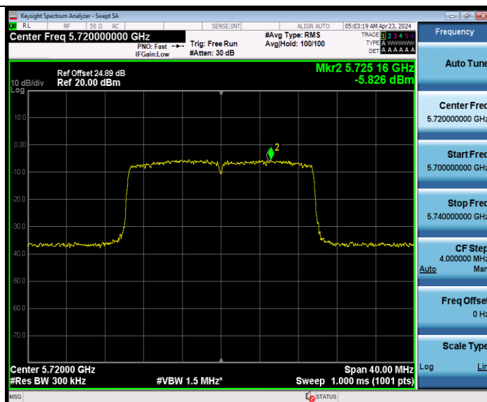
11AX20MIMO_Ant9_5720_UNII-3
