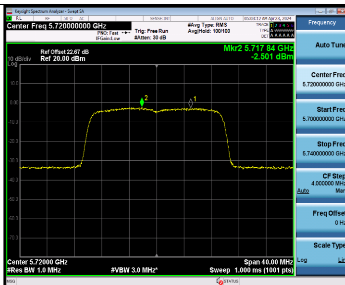
11AX20MIMO_Ant9_5720_UNII-2C
